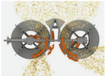
Distribuidor radial para un eficiente reparto de la paja con una mínima necesidad de fuerza
